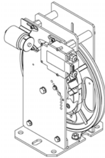
Abb. 2 Geschwindigkeitsbegrenzer Typ LK120/LX120/LX150/LX180/LX200 (bzw. LK200/LK250/LK300/LK315) mit Fernauslösung
