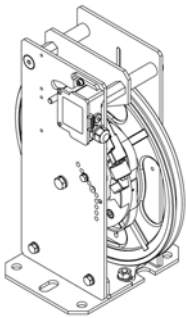
Abb. 1 Geschwindigkeitsbegrenzer Typ LK120/LX120/LX150/LX180/LX200/LK200 (bzw. LK250/LK300/LK315) ohne Fernauslösung
