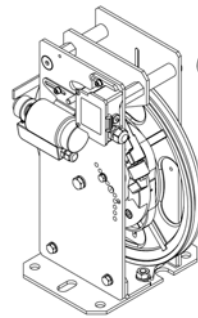
Abb. 3 Geschwindigkeitsbegrenzer Typ LK120/LX120/LX150/LX180/LX200 (bzw. LK200/LK250/LK300/LK315) mit Vorrichtung für unkontrollierte Bewegungen der Kabine
