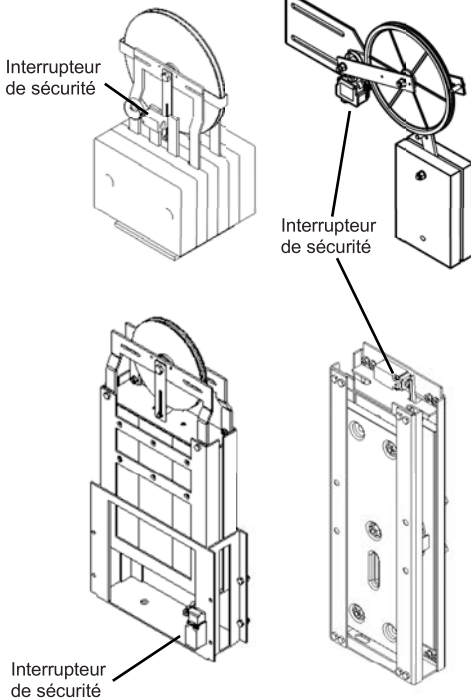
Fig. 5 Tendeur par contrepoids vertical doté d'interrupteur de sécurité
