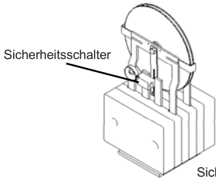
Abb. 1 Geschwindigkeitsbegrenzer Typ LK120/LX120/LX150/LX180/LX200/LK200 (bzw. LK250/LK300/LK315) ohne Fernauslösung
