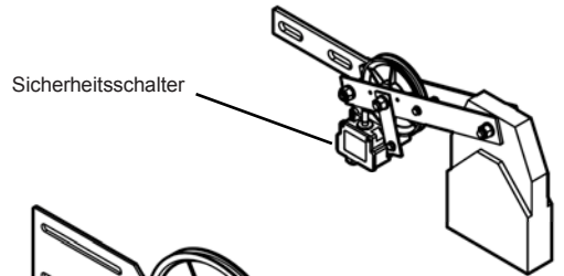
Abb. 3 Geschwindigkeitsbegrenzer Typ LK120/LX120/LX150/LX180/LX200 (bzw. LK200/LK250/LK300/LK315) mit Vorrichtung für unkontrollierte Bewegungen der Kabine
