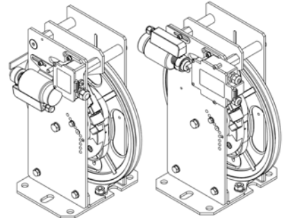
Fig. 3 Limiteur de vitesse Mod. LK120/LX150/LX180/ LK200/LK250/LK300/LK315 avec dispositif pour mouvement incontrôlé de la cabine
