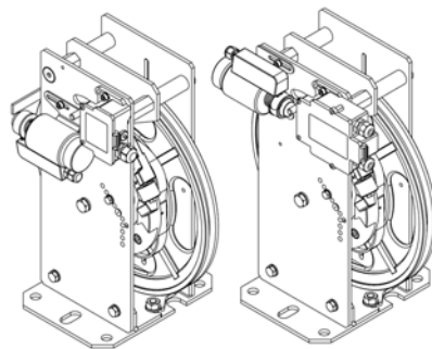
Fig. 3 Limitador de velocidad Mod. LK120/LX120/LX150/LX180/ LX200/ LK200/LK250/LK300 /LK315 con dispositivo para movimiento incontrolado de la cabina
