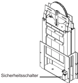
Abb. 5 Spanngewicht mit Senkrechtem Sicherheitsschalter
