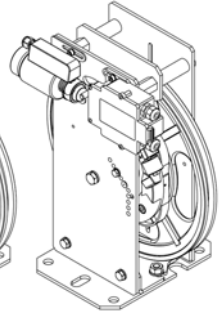
Abb. 3 Geschwindigkeitsbegrenzer Typ LK120/LX120/LX150/LX180/LX200 (bzw. LK200/LK250/LK300/LK315) mit Vorrichtung für unkontrollierte Bewegungen der Kabine
