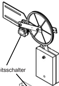
Abb. 2 Geschwindigkeitsbegrenzer Typ LK120/LX120/LX150/LX180/LX200 (bzw. LK200/LK250/LK300/LK315) mit Fernauslösung
